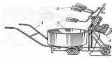
Рис. 5.2. Растворосмеситель: CO-23В: 1 — тележка; 2 — смесительный барабан; 3 — лопасть; 4 — электродвигатель
