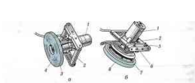
Рис. 5.15. Штукатурно-затирачные электрические машины: а – СД-88А, б – СД-112А; 1 – корпус электродвигателя; 2 – ручка; 3, 4 и 6 – затирачные диски; 5 – электронная кнопка; 6 – регулятор скорости; 7 – резиновый подвесок
