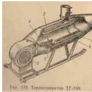
Рис. 170. Теплоагрегат ТТ-150:
